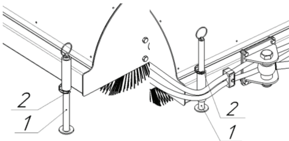
Рисунок 11 – Перемещение опорных стоек
