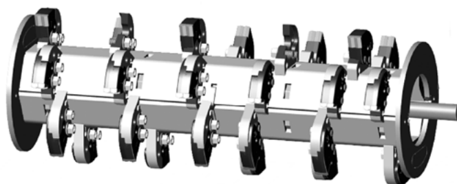
Ротор с фиксированными молотками с вольфрамовой напайкой
