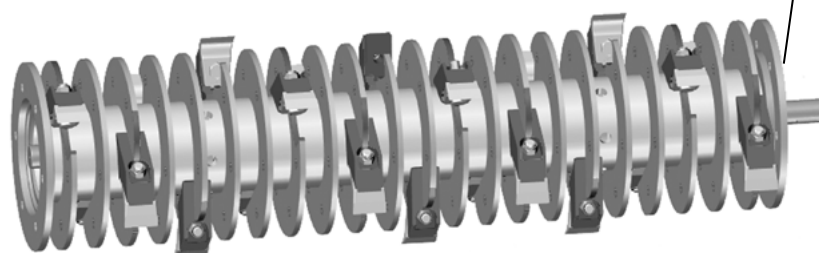
Ротор с фиксированными молотками с вольфрамовой напайкой
