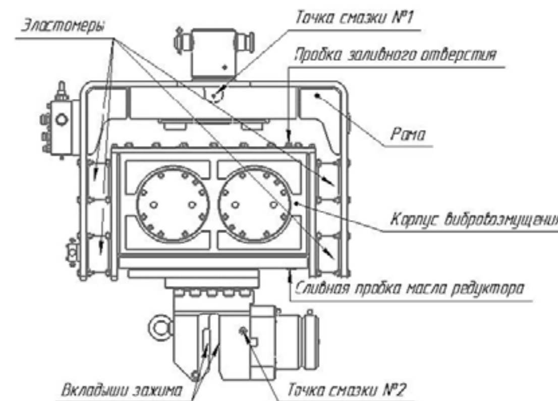
Рис. 5 Вибропогрузатель
