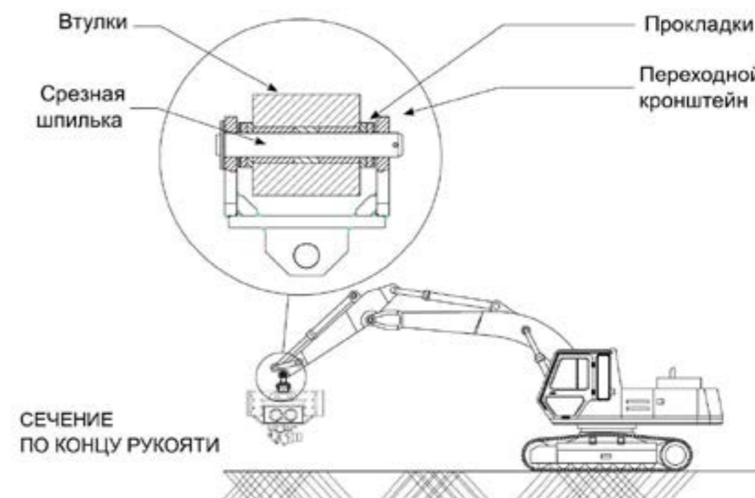
Рис. 6. Положение переходного адаптера на машине.
