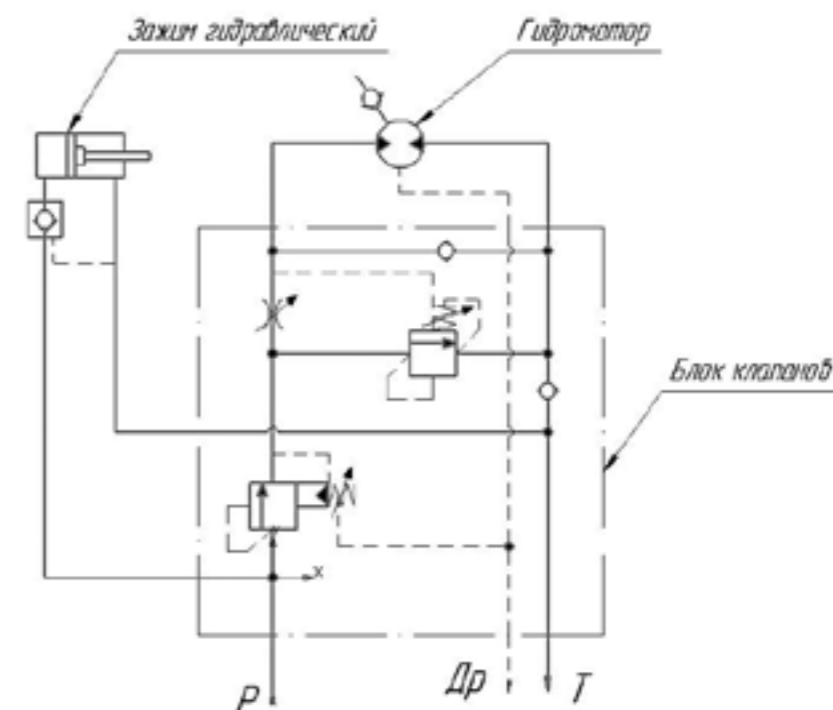
Рис. 8. Гидравлическая схема для вибропогрузателя VP 500
