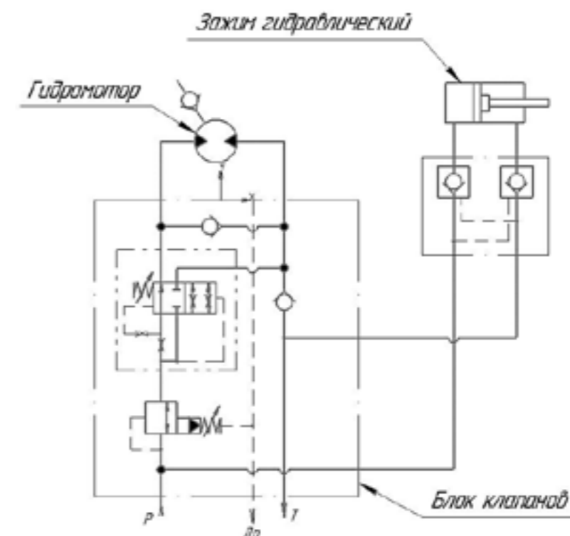
Рис. 7. Гидравлическая схема для вибропогрузателя VP 310
